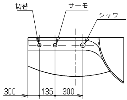
水栓取付け位置 (フリー)
